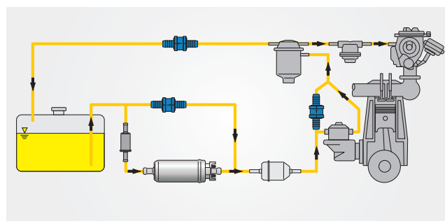
Ejemplo de aplicación: Motor de carburador con bomba adicional eléctrica conmutable
